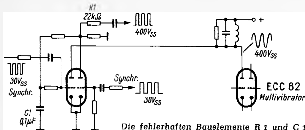
Die fehlerhaften Bauelemente R 1 und C 1 verursachen einen viel zu hohen Stromfluß durch das erste Triodensystem
