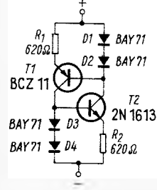
Bild 3. Diese Schaltung arbeitet ähnlich der von Bild 1. Der Arbeitsbereich beginnt jedoch schon bei 1,8 V
