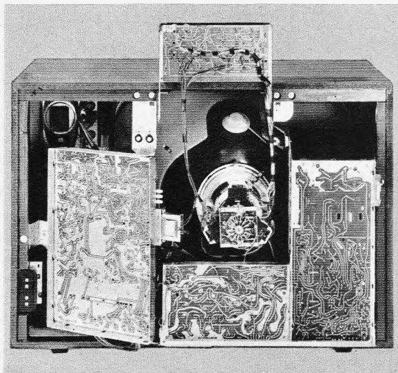
Links: Bild 7. Servicefreundliches Farbfernsehgeräte-Chassis. Links die Chromplatte als Schwenkchassis, oben die ausklappbare Konvergenz-Platine und rechts das L-förmige Klappchassis mit Leiterplatten für Ablenkung und Hochspannungserzeugung (Werkaufnahme: Metz)
