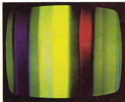
Bild F 11. Phasenbalkentestbild bei verstimmter Durchlaßkurve des Bild-Zf-Verstärkers
