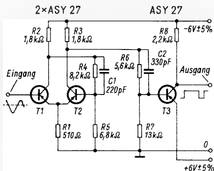
Schaltung des Schmitt-Triggers für Impulsfolgefrequenzen bis 100 kHz
