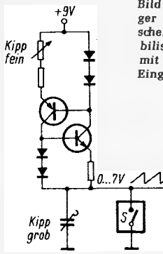
Bild 10. Linearisierung eines Oszillografenkippteiles mit elektronischer Drossel. Der Konstantstrom ist einstellbar
