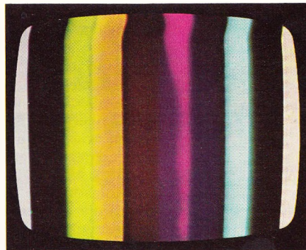
Bild F 9. Phasenbalkentestbild bei Übersteuerung des Zf-Verstärkers
