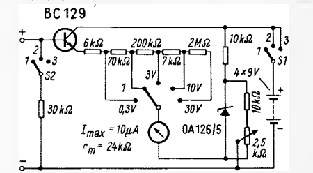
Bild 3. Die vollständige Schaltung des Gleichspannungs-Transistorvoltmeters nach Telefunken-Unterlagen
