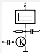
Bild 8. Elektronische Drossel als Kollektorstromwiderstand
