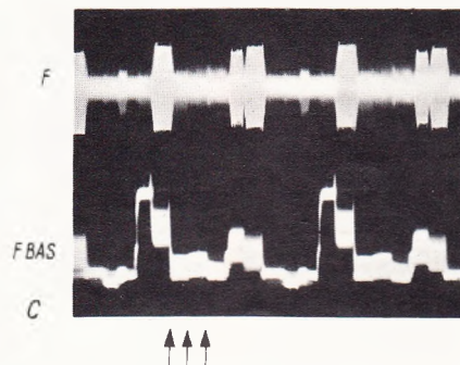
Bild 12c. FBAS- sowie F-Signal mit begrenzten Synchronimpulsen sowie begrenzten Amplituden der Farbartsignale Rot, Purpur und Blau
