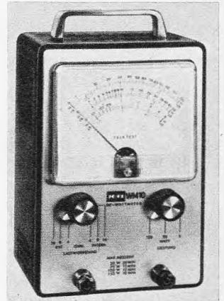
Nf-Wattmeter, Typ WM 10 (Werkbild: Klein + Hummel)
