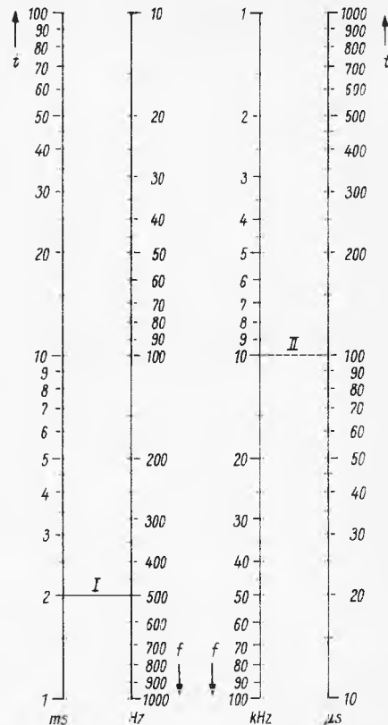
Nomogramm zum Ermitteln der entsprechenden Zeit aus einer Frequenz und umgekehrt
