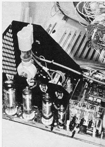
Links: Bild 3. Burggraf Color 1045 mit zwölf Röhren, 41 Transistoren, 45 Dioden und vier Gleichrichtern (Werkaufnahme: Graetz)
