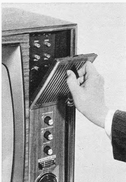
Bild 5. Die Konvergenzplatte steckt hinter dem abnehmbaren Hochtonlautsprecher (Werkaufnahme: Grundig)
