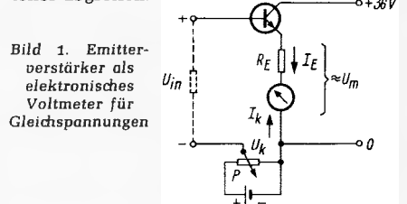
Bild 1. Emitterverstärker als elektronisches Voltmeter für Gleichspannungen
