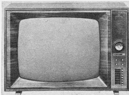
Bild 11. Farbfernsehempfänger Bildmeister FF 91 (Werkaufnahme: Siemens)
