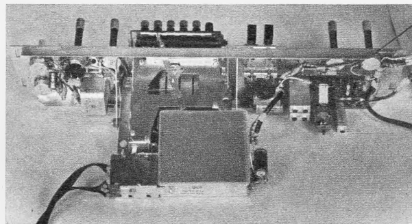
Bild 5. Bedienfeld-Einschub mit Kanalwähler und erster Zf-Stufe. Gegenüber einem Schwarzweißempfänger kommen folgende Bedienelemente hinzu: Farbsättigungseinsteller, Farbtonblende und Taste Farbe/Schwarzweiß (zur Demonstration gedacht, da der Farbschalter automatisch arbeitet)
