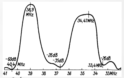
Bild 7. Zf-Durchlaßkurve am Farbgleichrichter
