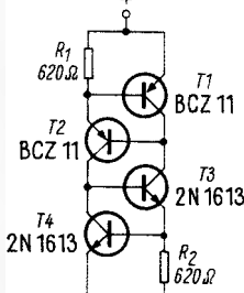
Bild 2. Elektronische Drossel mit einem Arbeitsbereich ab 1,8 V
