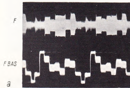
Links: Bild 12a. FBAS- sowie F-Signal einer nach dem Phasenwinkel geordneten Farbbalken- folge am Ausgang des Leuchtdichtegleich- richters
