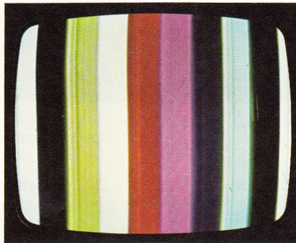
Bild F 18 Phasenbalkentestbild mit Überschwingen durch Reflexionen bei nicht abgeschlossener Verzögerungsleitung
