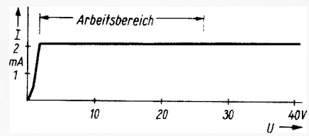
Bild 6. Kennlinie der Schaltung in Bild 3
