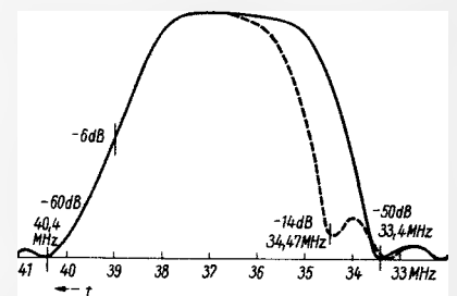
Bild 6. Zf-Durchlaßkurve am Leuchtdichte-Gleichrichter
