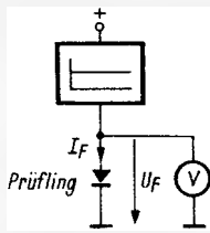
Bild 9. Konstantstromquelle zur Messung der Vorwärtsspannung von Dioden
