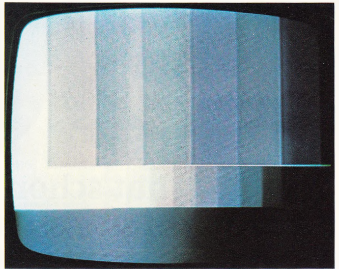
Bild F 2. Leuchtdichtesignalbild einer helligkeitsgeordneten Farbbalkenfolge, sog. Treppenkantenfolge
