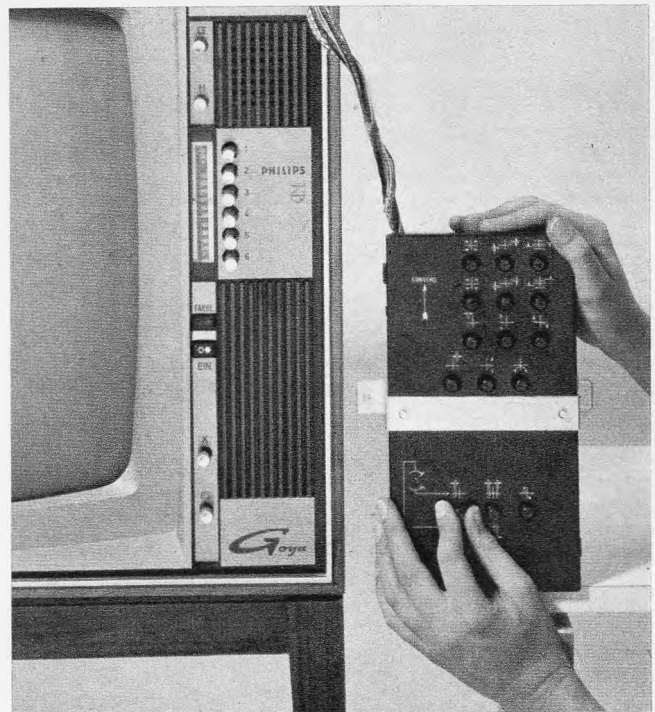
Bild 9. Konvergenzeinheit zum Einstellen der Trimmwiderstände, aus dem Gehäuse herausgenommen
