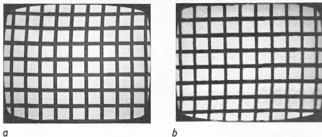
Bild 11. Schirmbilder bei Einspeisen eines Zf-Signals an den einzelnen Meßpunkten eines Bild-Zf-Verstärkers: a = 50 mV am Meßpunkt 7, 10 mV am Meßpunkt 6; b = 10 mV am Meßpunkt 5
