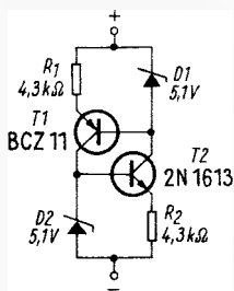
Bild 1. Elektronische Drossel mit einem Arbeitsbereich von 9...35 V
